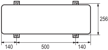
Dimensiones para fijar la unidad externa al piso. Unidades en mm Sistemas de 9 000 BTU/h, 12 000 BTU/h y 18 000 BTU/h de capacidad
