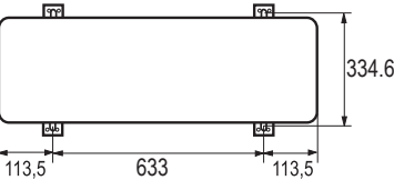
Dimensiones para fijar la unidad externa al piso. Unidades en mm Sistemas de 24 000 BTU/h de capacidad
